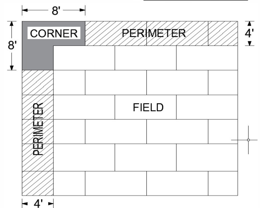
ASCE 7-10, h \geq 60' FT
